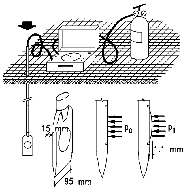
Figura 1 - Prova DMT: schema di funzionamento
