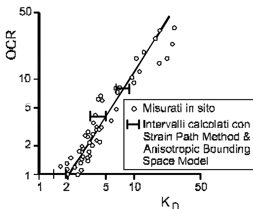
Figura 6 - Correlazione teorica K_D - OCR (Finno, 1993)
